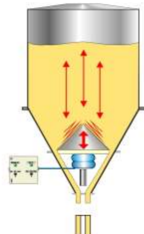
Getakteter Austrag: Ventil pulsiert auf und ab und vibriert
