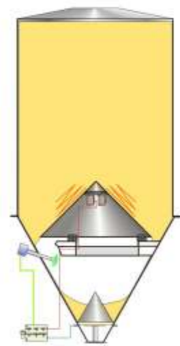
Füllstandssonde aktiviert oberes Ventil, Austragstrichter wird befüllt
