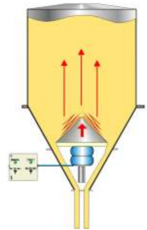
Kontinuierlicher Austrag: Ventil hebt sich und vibriert
