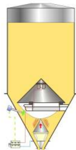
Füllstandssonde aktiviert oberes Ventil, Austragstrichter wird befüllt
