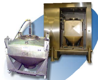
IBC 清洗机
